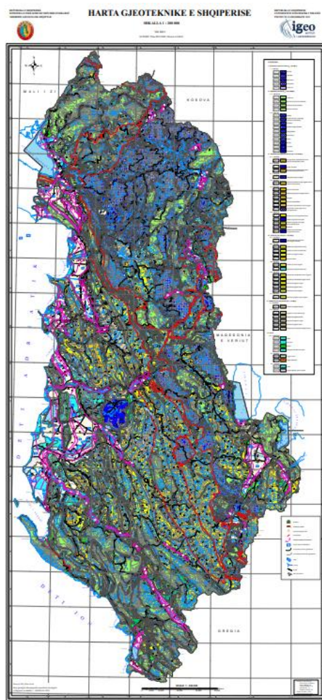
Figura 1 Harta Gjeoteknike e Shqipërisë
